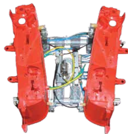
Mani di presa per stampaggio plastica
