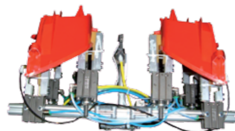
Mani di presa per stampaggio plastica
